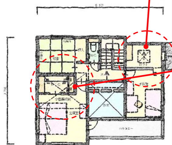
2階平面図
